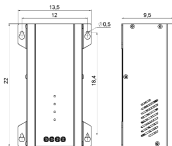
Figura 10 – Dimensões
