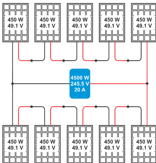
Figura 8 - Instalação de Placas Fotovoltaicas.
