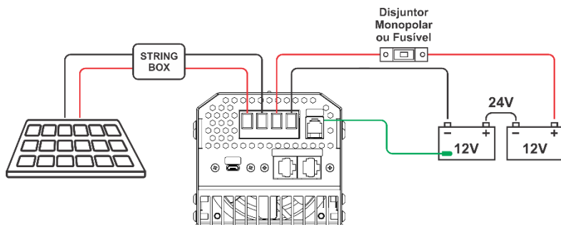
Figura 7 - Esquema de Ligação.
