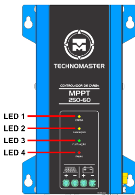
Figura 2 – Vista Frontal.
