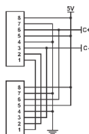
Figura 1 – Pinagem RJ45.
