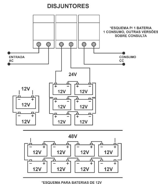
Figura 2 – Esquema de ligação.
